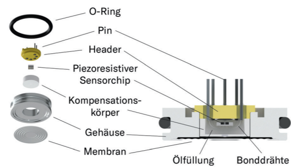
Abbildung 2: Aufbau eines isolierten, ölgefüllten piezoresistiven Drucksensors.
