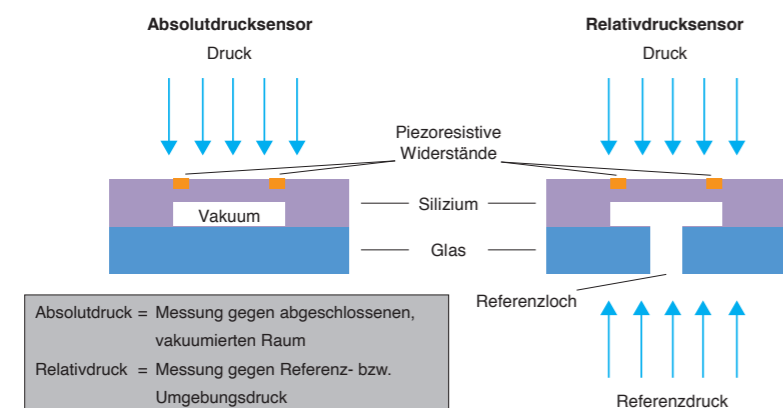
Abbildung 1: Aufbau des piezoresistiven Sensorchips.
